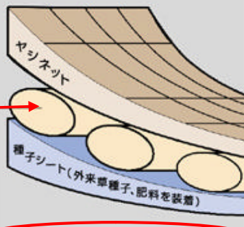
基材袋(植生基材、在来・木本類種子、肥料を封入)
